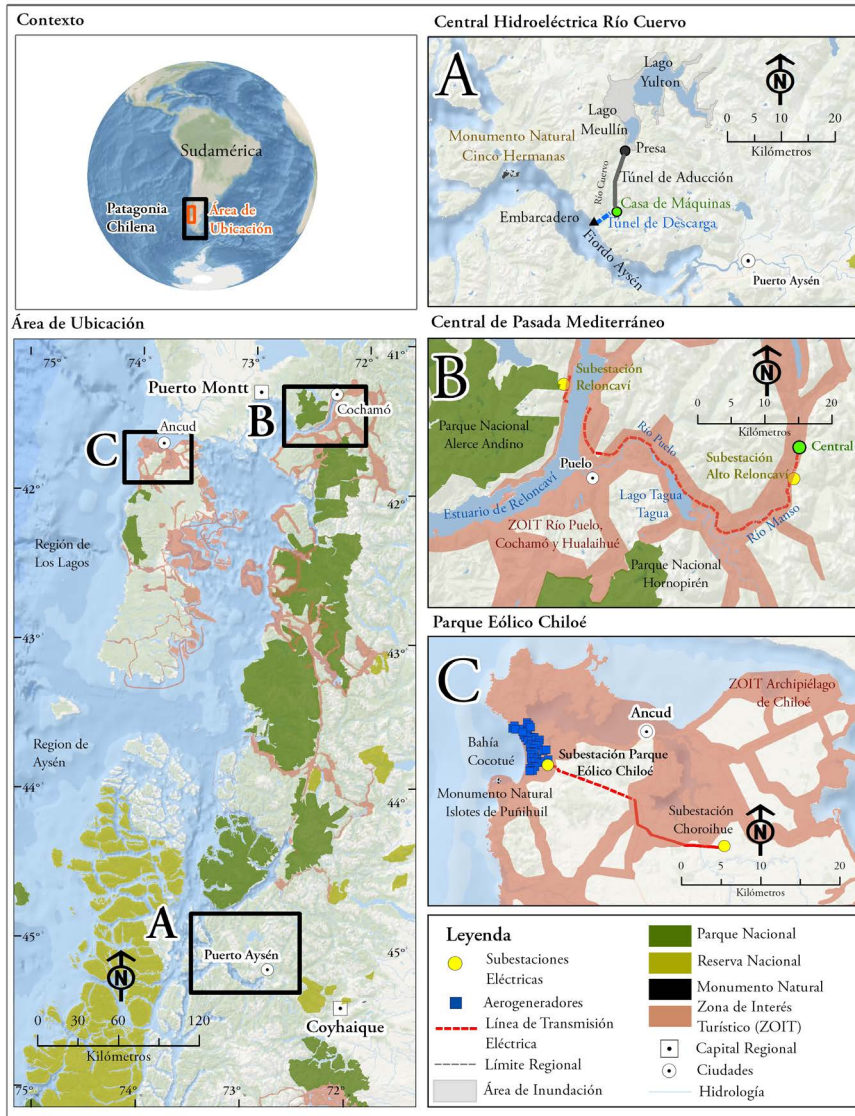
FIGURA 1 | Ubicación y características de los proyectos energéticos
